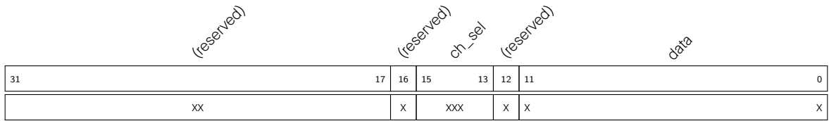
图 36-9. GDMA 数据格式
