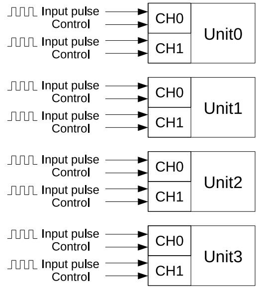
图 29-1. PCNT 框图
