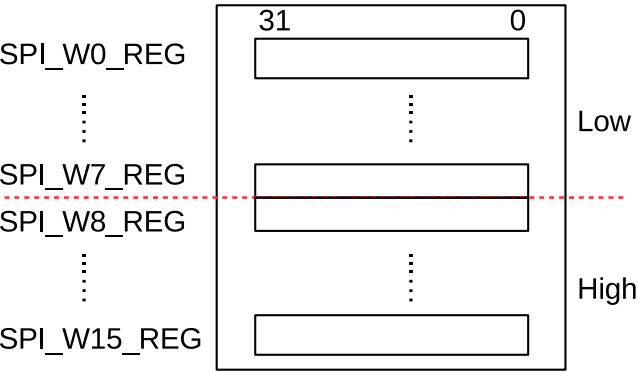
图 26-2. CPU 控制的传输中使用的数据 Buffer
