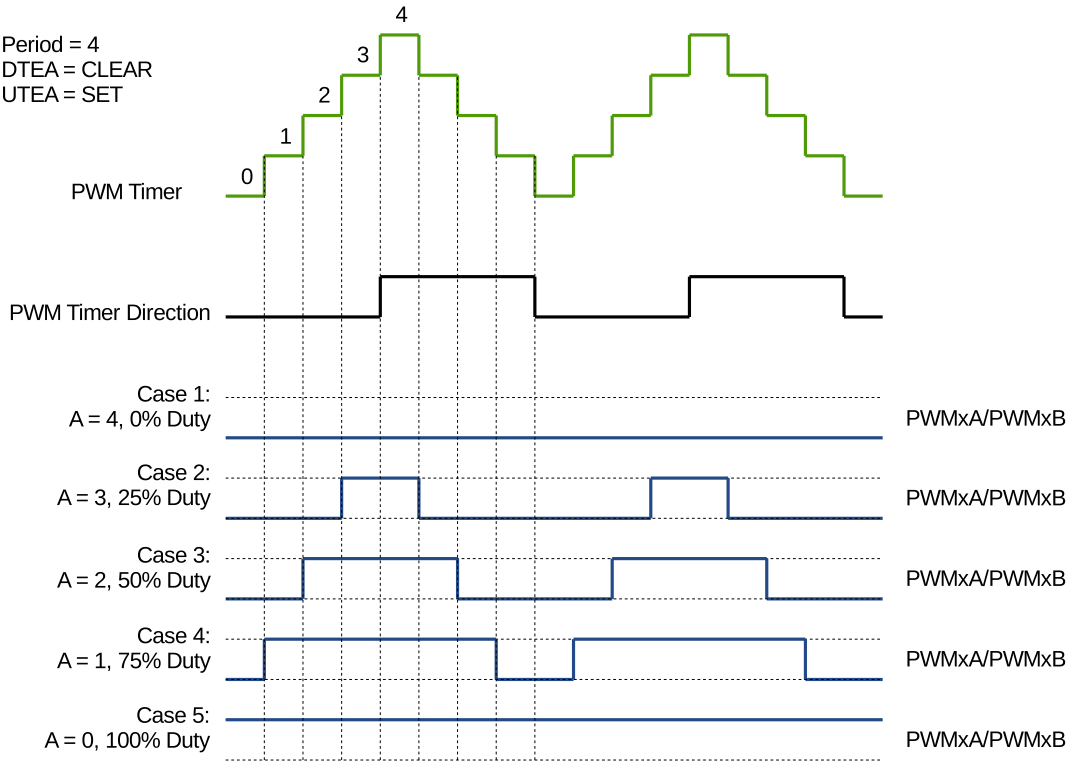
图 33-16. 递增递减模式下的对称波形
