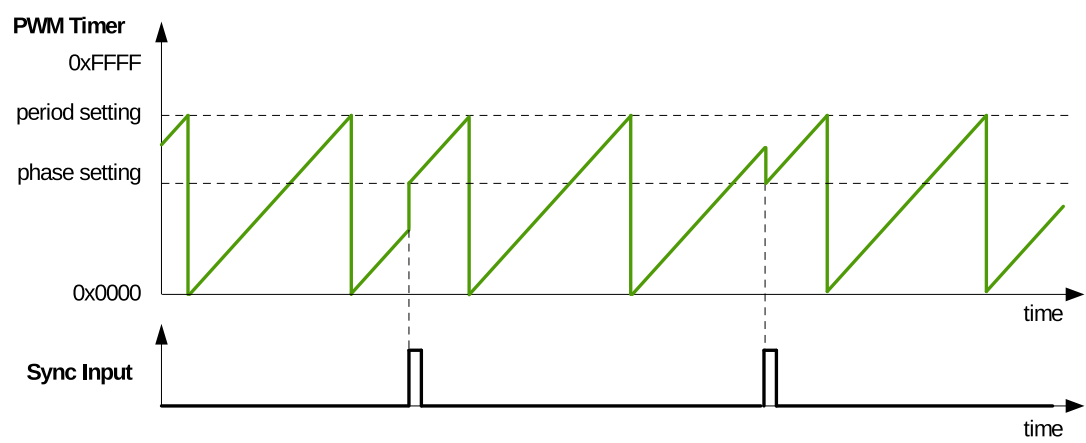
图 33-8. 递增计数模式波形
