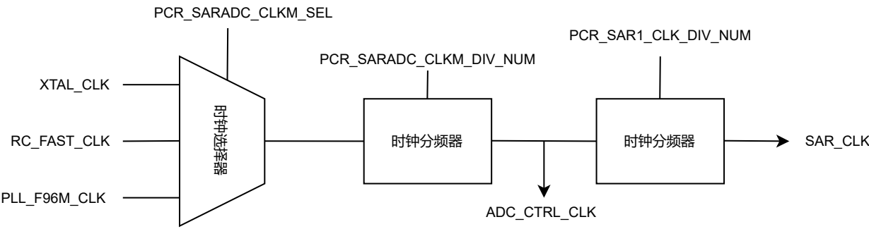
图 36-2. SAR ADC 时钟结构图
