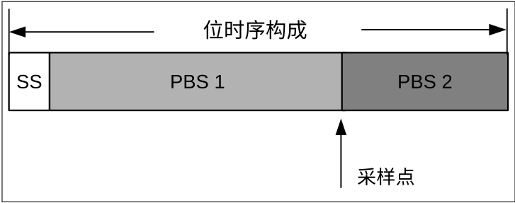
图 31-5. 标称位构成
