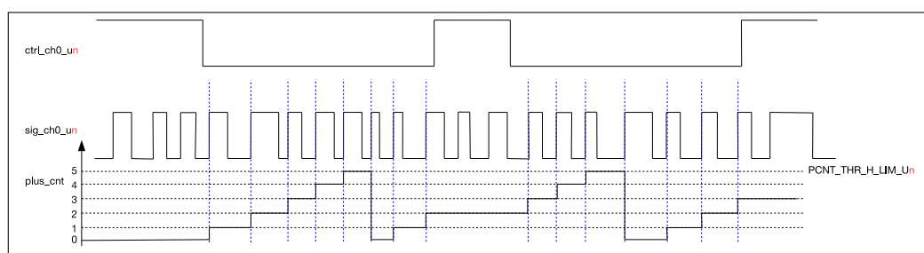
图 29-3. 通道 0 递增计数图
