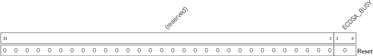
Register 23.8. ECDSA_STATE_REG (0×0020)
