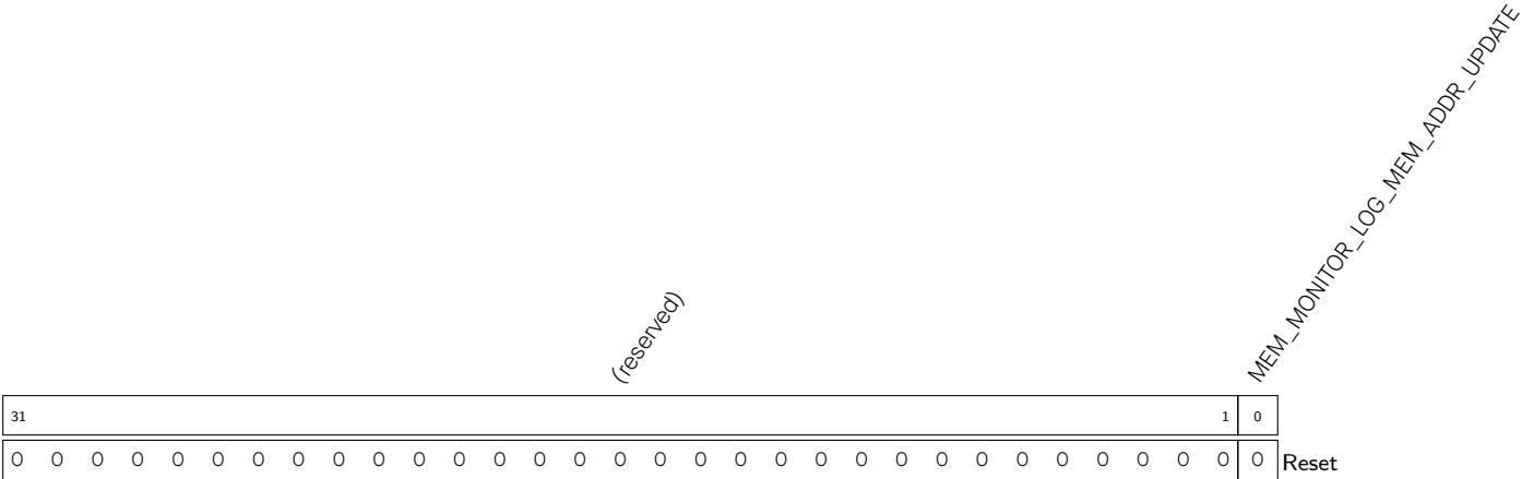
Register 16.9. MEM_MONITOR_LOG_MEM_ADDR_UPDATE_REG (0×0020)
