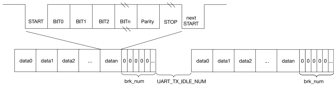
图 25-4. UART 数据帧结构
