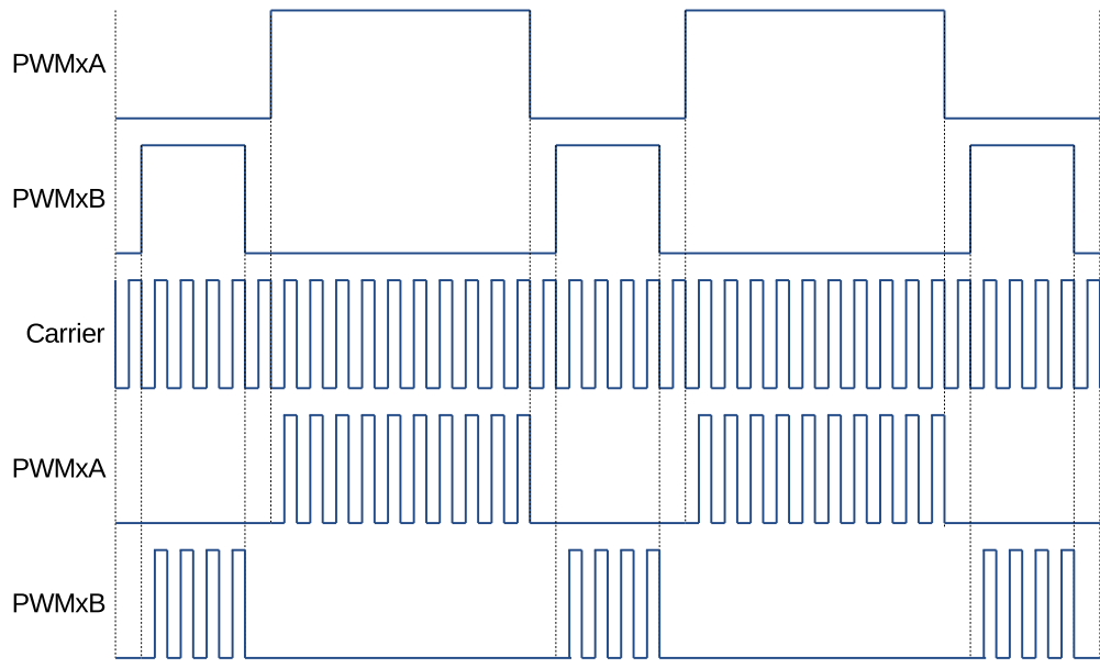
图 33-29. PWM 载波操作的波形示例
