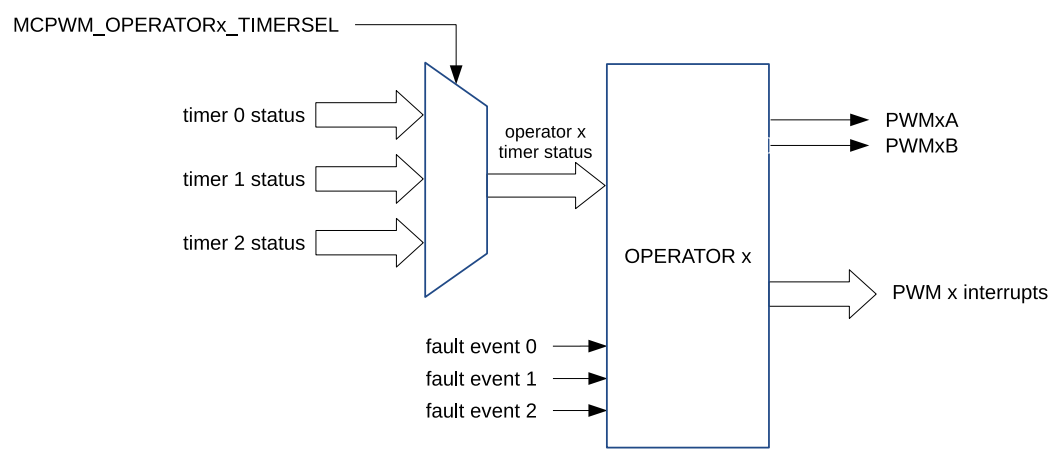
图 33-4. 操作器模块
