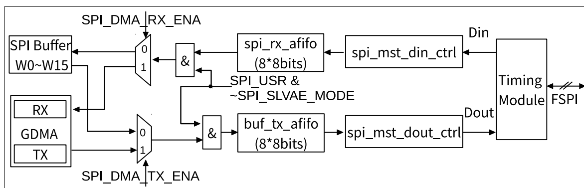
图 26-4. GP-SPI2 用作主机时的数据流控制
