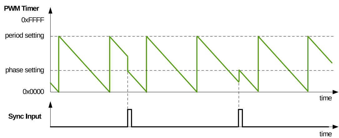
图 33-9. 递减计数模式波形
