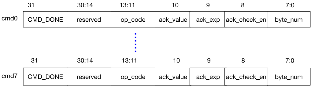
图 27-5. I2C 命令寄存器结构
