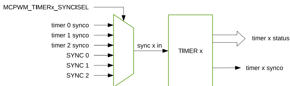
图 33-3. 定时器模块
