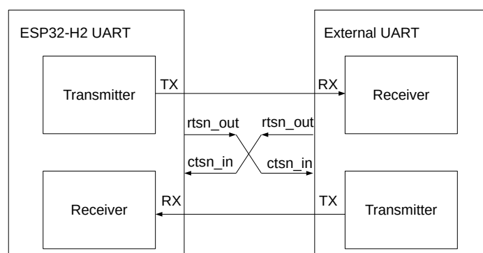
图 25-10. 硬件流控信号连接图
