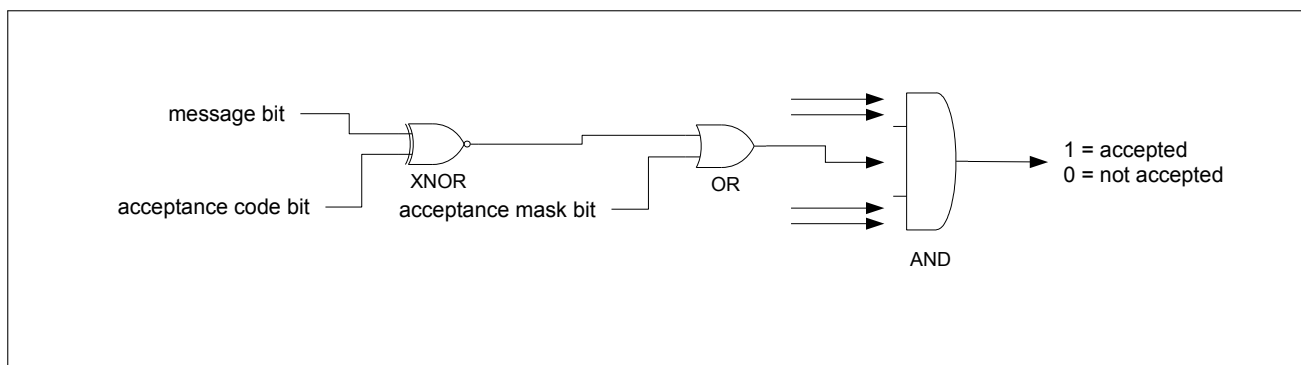
图 31-8. 接收滤波器
