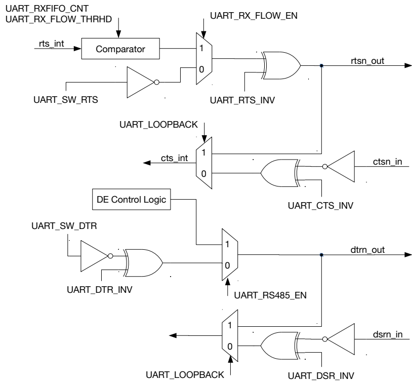
图 25-9. 硬件流控图
