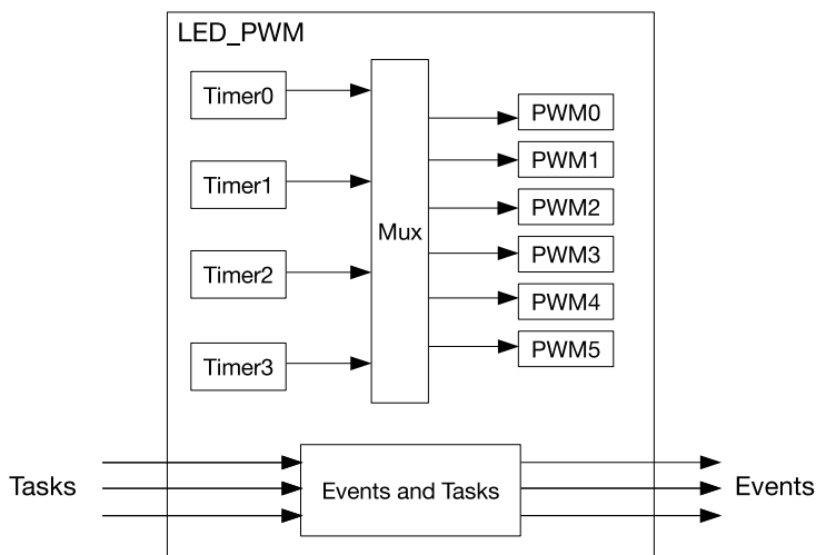
图 32-1. LED PWM 控制器架构
