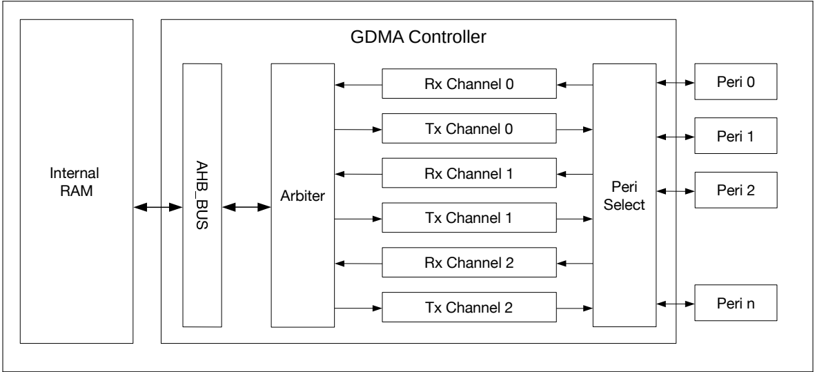
图 3-2. GDMA 控制器的架构
