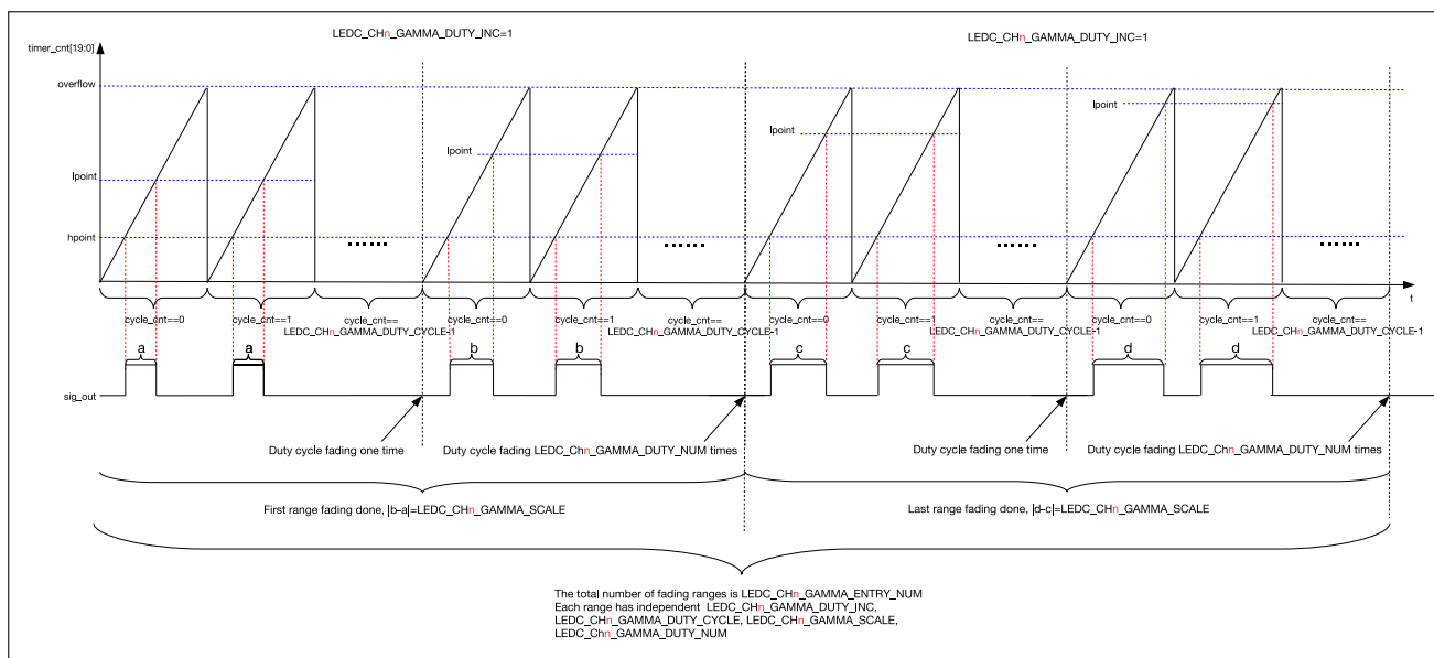
图 32-7. 输出信号占空比伽玛曲线渐变图
