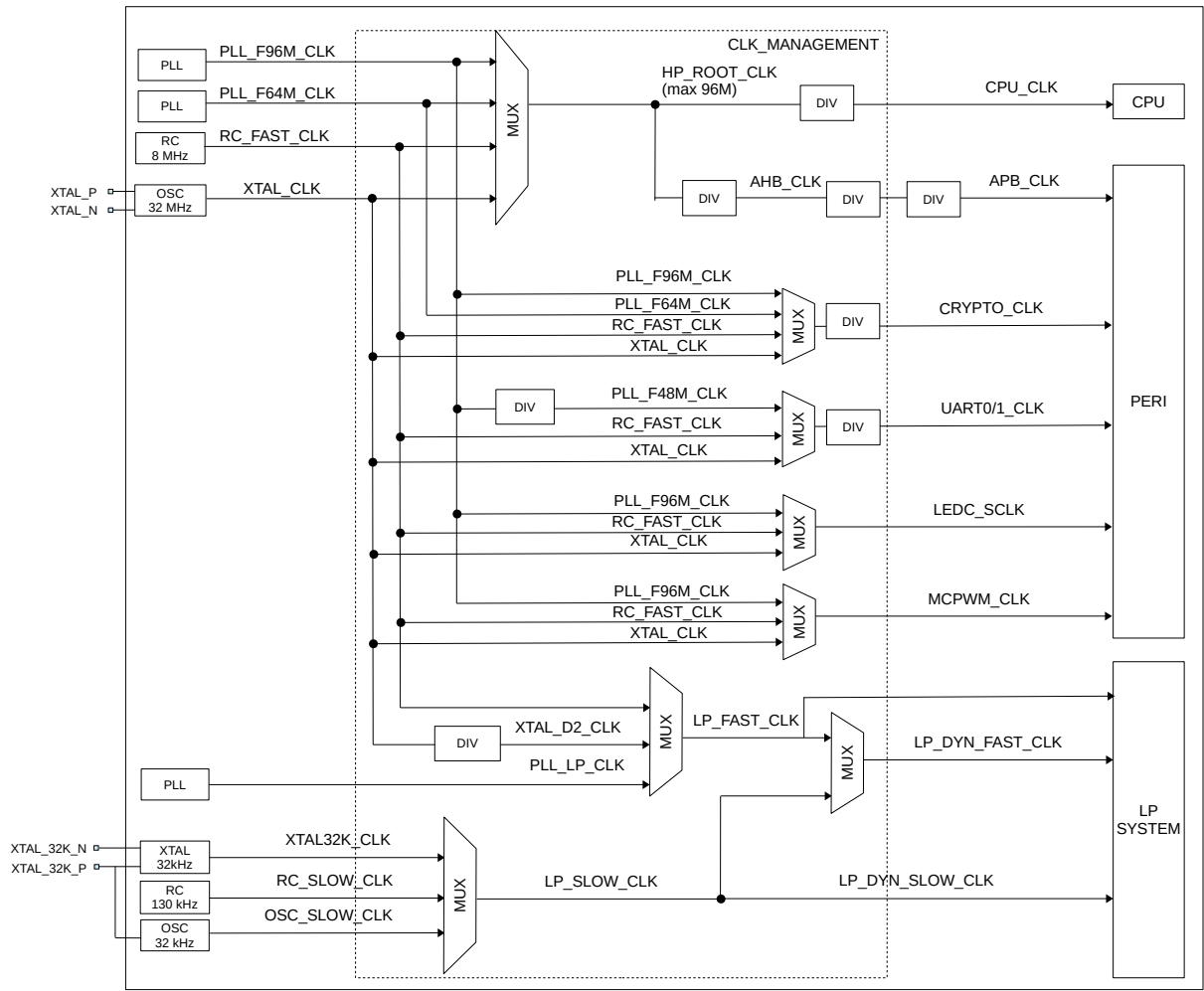
图 7-2. 系统时钟
