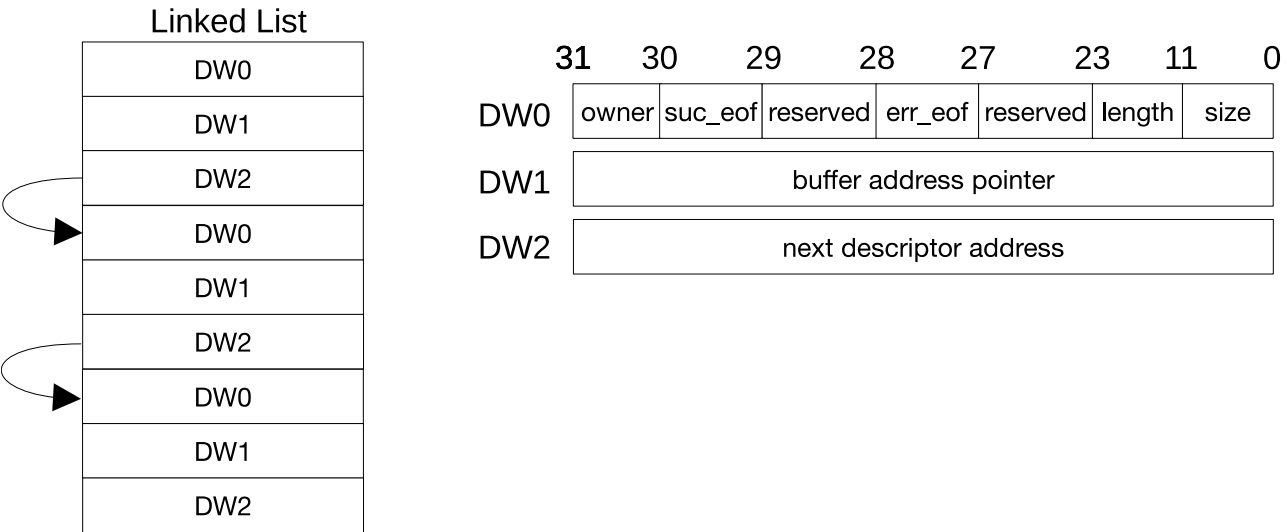
图 3-3. 链表结构图
