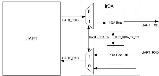
图 25-8. IrDA 编解码结构图
