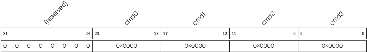
图 36-4. APB_SARADC_SAR_PATT_TAB1_REG 包含样式 0 - 3
