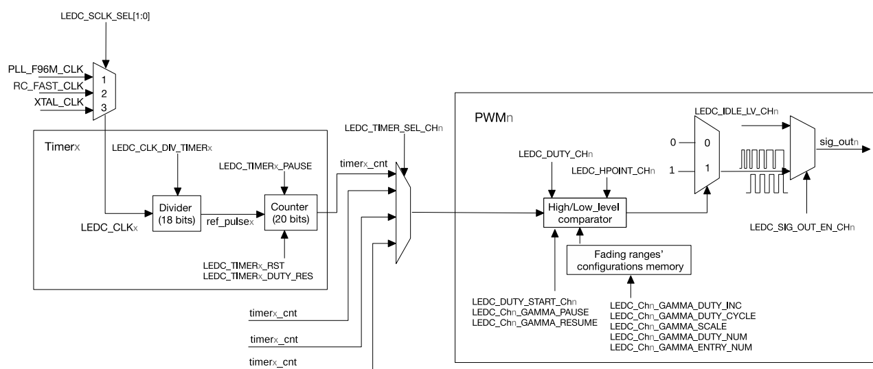
图 32-2. 定时器和 PWM 生成器功能框图
