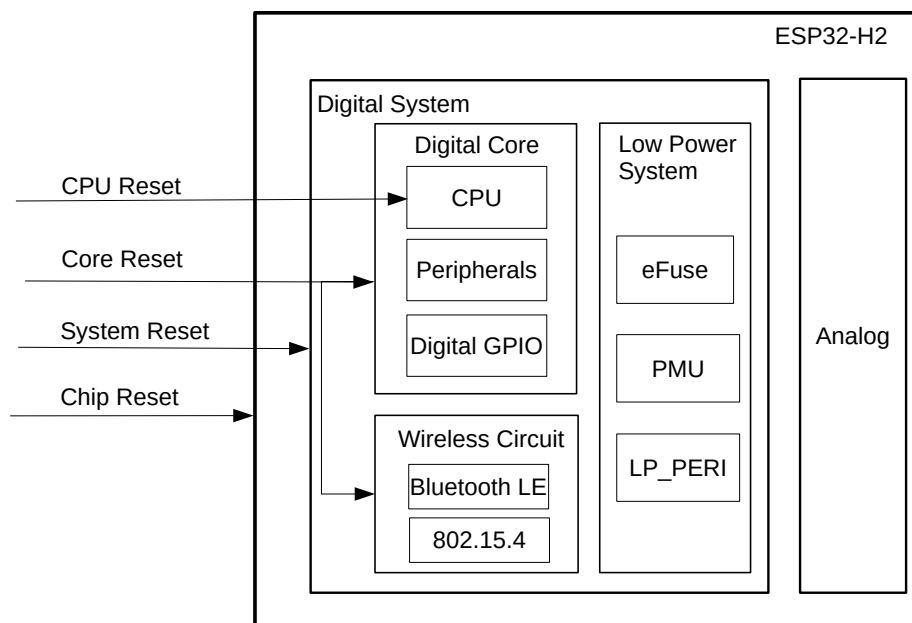
图 7-1. 四种复位等级
