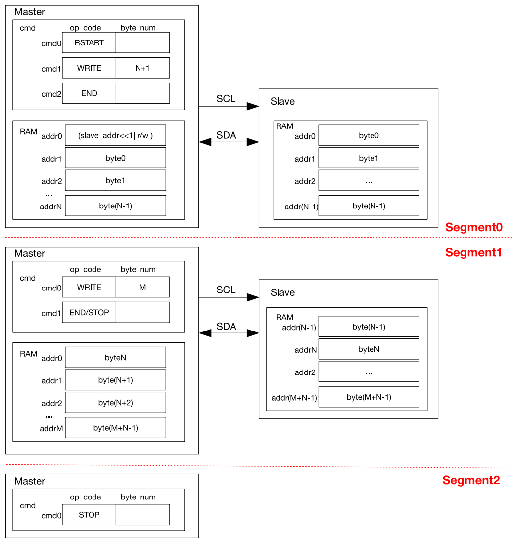
图 27-9. I2C 主机分段写 7 位寻址的从机
