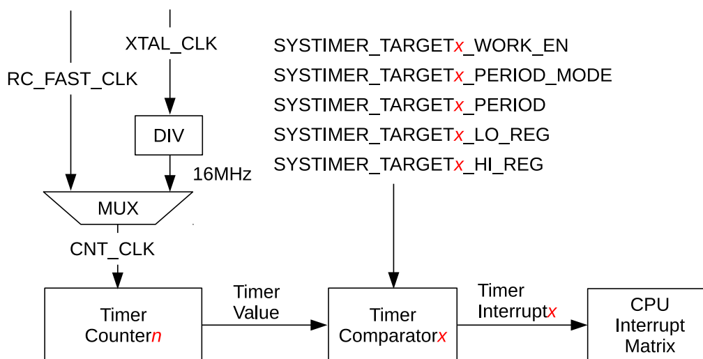
图 11-2. 系统定时器生成报警
