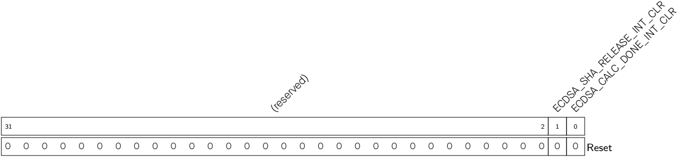
Register 23.7. ECDSA_INT_CLR_REG (0×0018)
