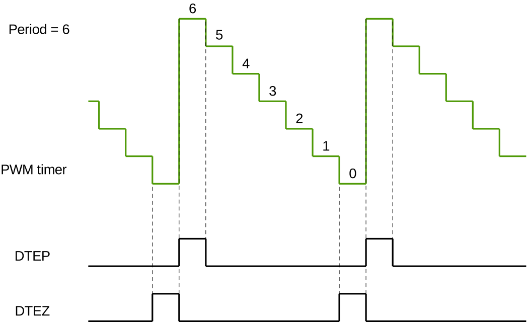
图 33-13. 递减模式中生成的 DTEP 和 DTEZ
