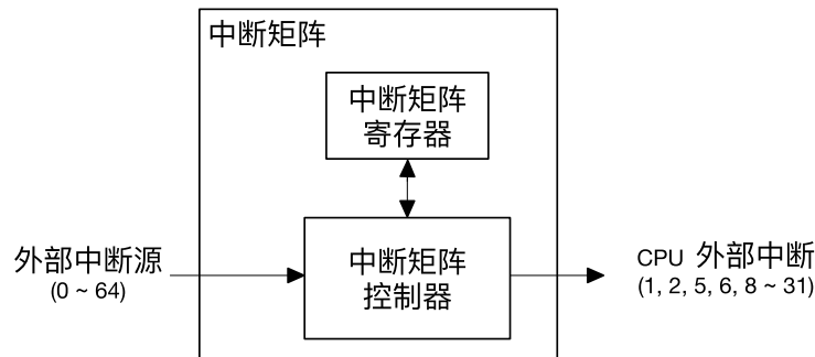
图 9-2. 中断矩阵结构图
